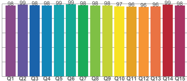
CQS: 97.5
