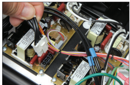
7) Install lamp output connector.
